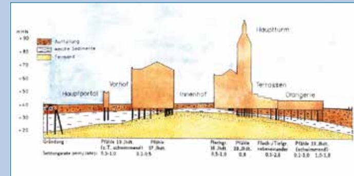
Abb. 6: Über dem eiszeitlichen Sandrücken bildete sich in der letzten Eiszeit eine weiche organische Schicht. Durch die Besiedlung der Insel sammelte sich darüber eine Auffüllung aus überwiegend Sand und Bauschutt. Ausreichend tragfähig ist allein der Sandrücken.
